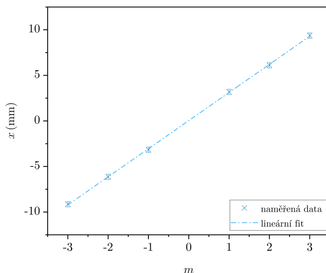
Graf 10: Závislost polohy difrakčních minim x na jejich řádu m pro difrakci na dvojštěrbíně B
